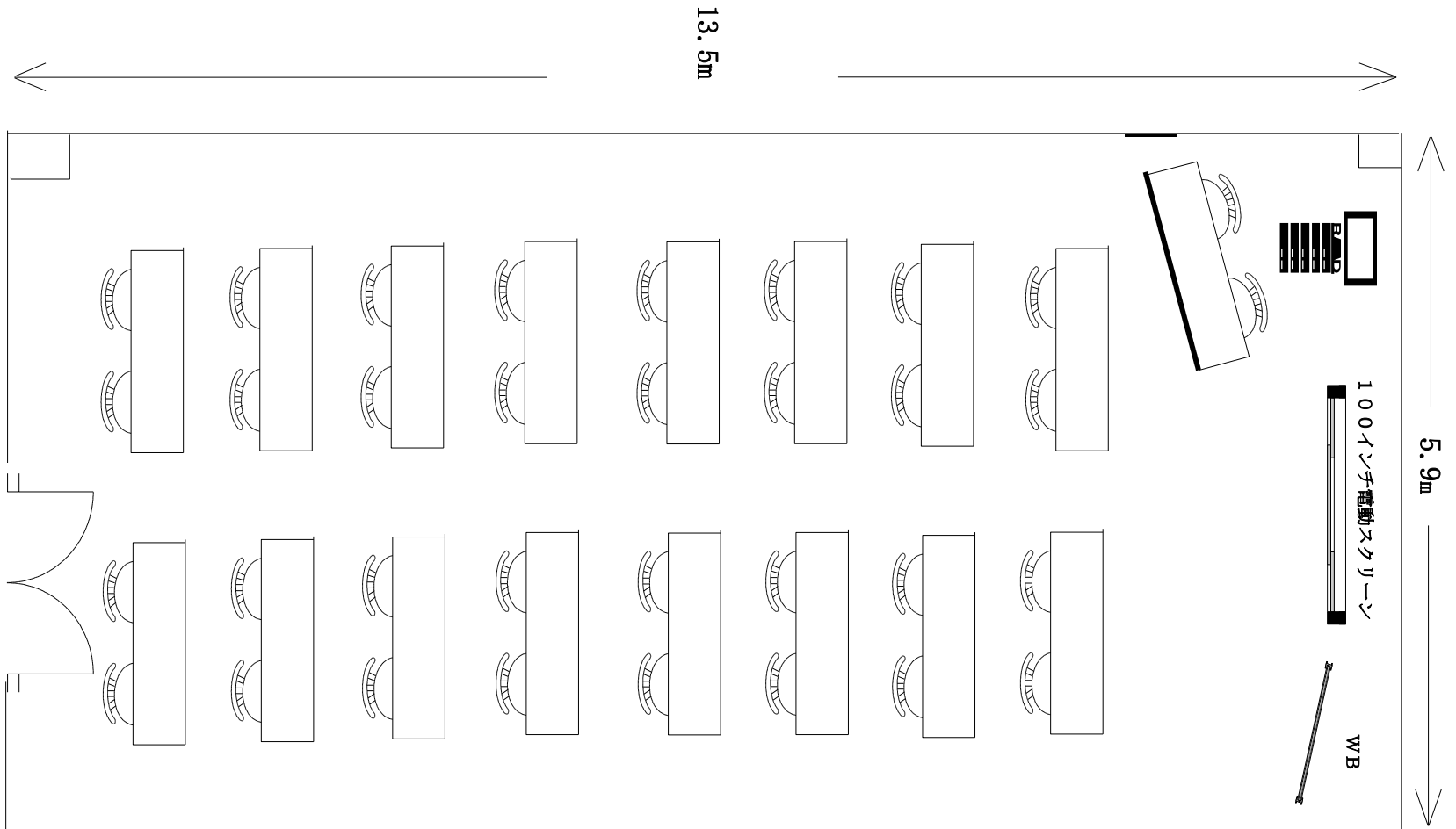
4 F 第2会議室配置図 (教室型) (75.0m 2 )
